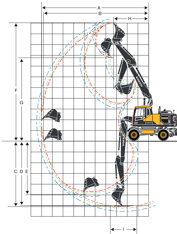
2-teiliger Ausleger 5.72 m und Aushubarm 2.45 m, 2.6 m, 2.9 m
