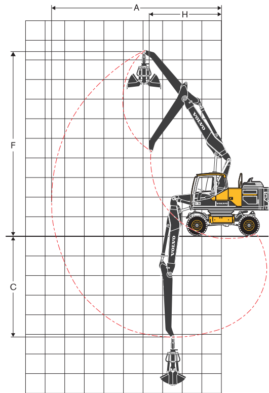
2-teiliger Ausleger 5.47 m und Aushubarm 3.2 m
